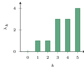
Espectro \lambda_k
