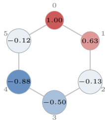
Reconstrucción k = 4 modos
