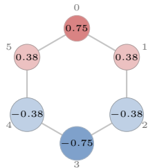
Reconstrucción k = 2 modos
