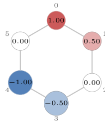
Reconstrucción completa ( k = 6 )
