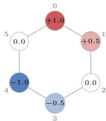
Señal f en C_6
