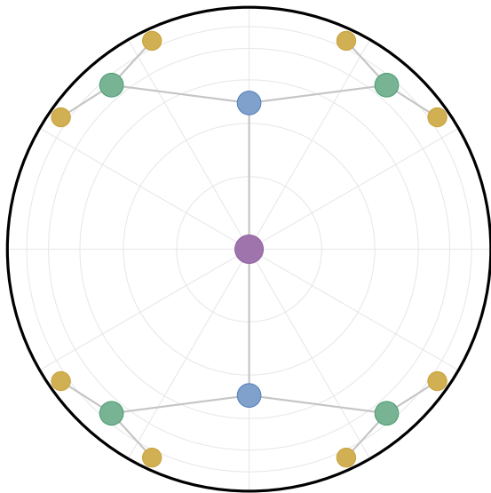
Embedding en disco de Poincaré
