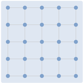
Euclidiano
