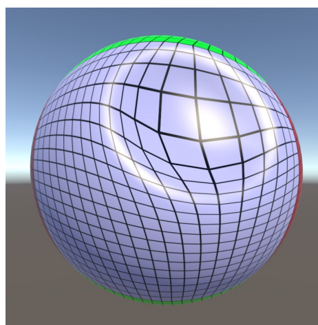
Figura 3: "Sfera" deformata
