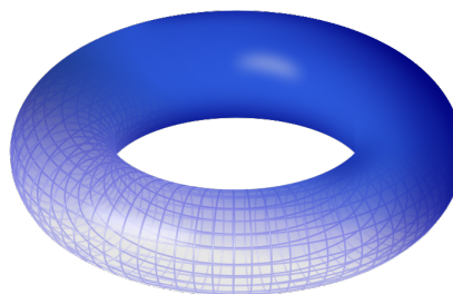
Figura 8: Toro
