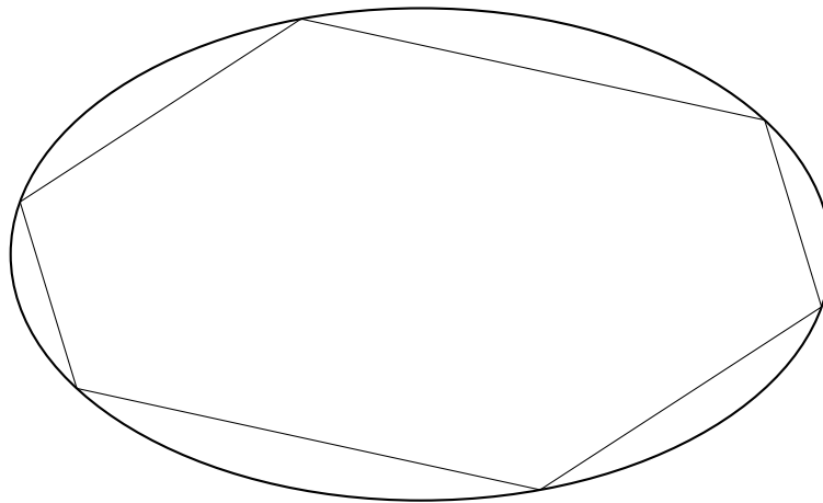
Figura 5: Orbita di periodo 6
