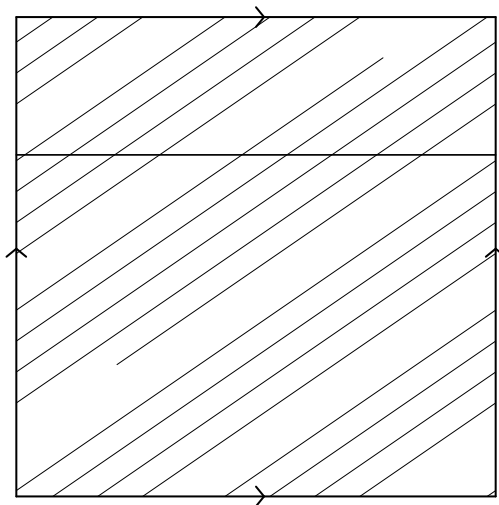
Figura 8: Flusso sul toro
