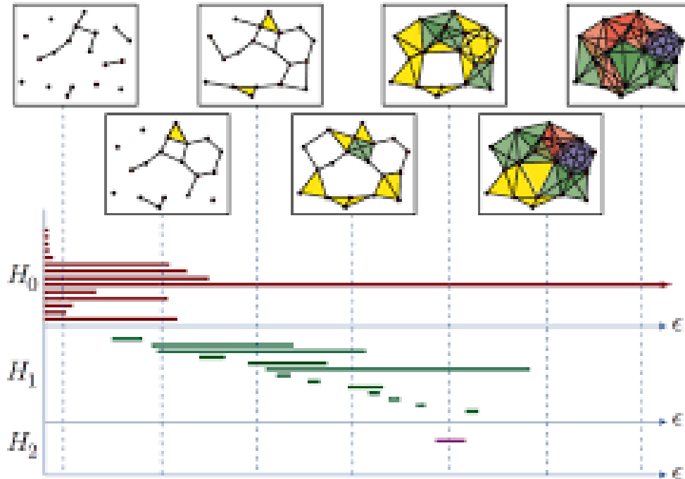
Figura 15: Un esempio di barcode per la successione di complessi di Rips costruita precedentemente
