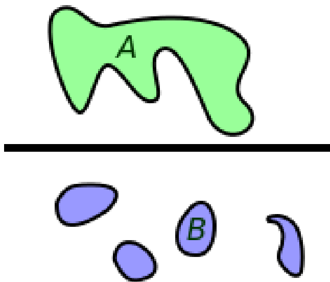
Figura 6: Due diversi spazi topologici
