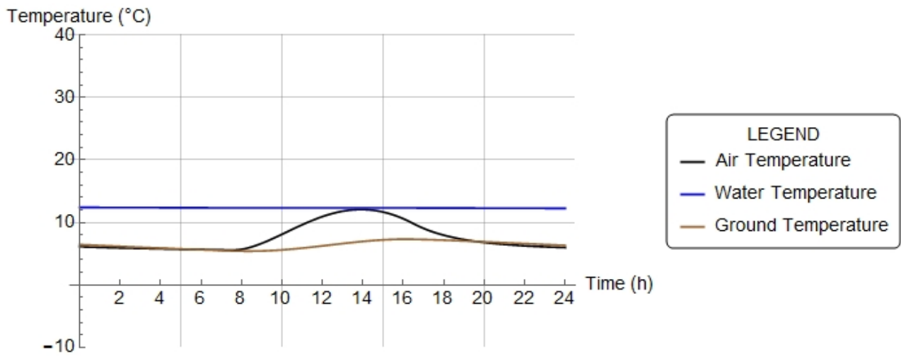
(d) Winter Solstice
