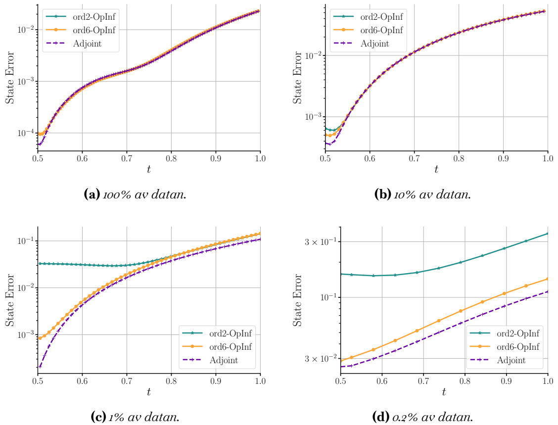
Figur 4.3: Prediktionsfel mot tid för varje körning av datadensitetsreducering i experimentet med Burgers ekvation.
