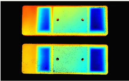
Zweiblock-Bahnschwellen – Blockgeometrie – Höhenkarte
