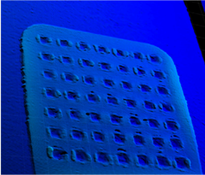
Schweißnähte am Zellkontaktersystem – Nahthöhe und -profil – Höhenkarte
