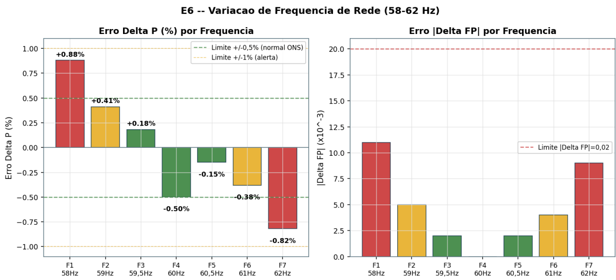
Figura 8 – Erro \Delta P(\%) (esquerda) e |\Delta FP| (direita) por nível de frequência de rede. Cores indicam a condição ONS: verde = normal, laranja = alerta, vermelho = emergência.
