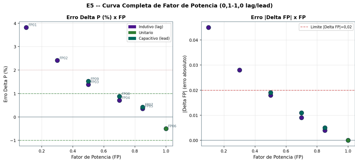
Figura 7 – Curva completa de FP: \Delta P(\%) \times FP (esquerda) e |\Delta FP| \times FP (direita) para os quadrantes indutivo, unitário e capacitivo.
