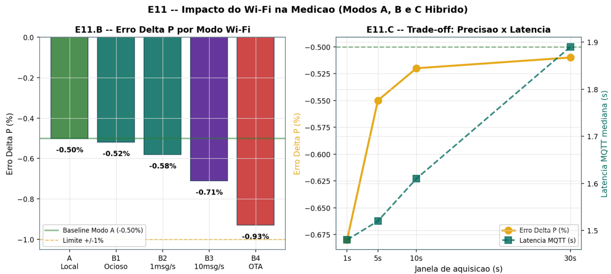
Figura 9 – Esquerda: \Delta P(\%) por modo Wi-Fi (A, B1–B4). Direita: trade-off entre erro \Delta P(\%) e latência MQTT em função da janela de aquisição no modo híbrido C.
