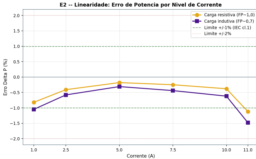
Figura 4 – Curva de linearidade: erro \Delta P(\%) em função da corrente para carga resistiva e carga indutiva. Linhas tracejadas indicam os limites de \pm 1\% e \pm 2\% .
