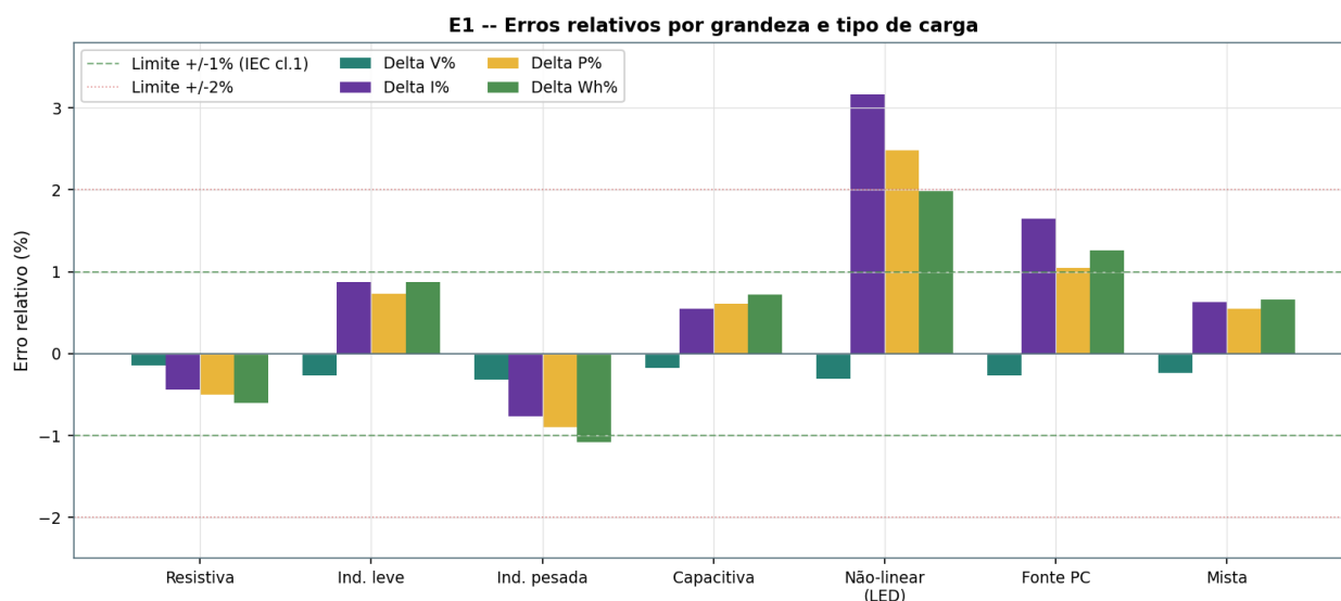
Figura 1 – Erros relativos \Delta V\% , \Delta I\% , \Delta P\% e \Delta Wh\% por tipo de carga. Linhas verdes indicam o limite de \pm 1\% (IEC 62053-21, classe 1); linhas vermelhas indicam o limite de \pm 2\% .
