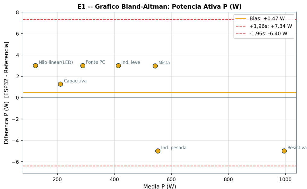
Figura 2 – Gráfico Bland-Altman: diferença entre as leituras ESP32 e referência em função da média das duas leituras. Linha amarela = bias ; linhas vermelhas = limites \pm 1,96\sigma .
