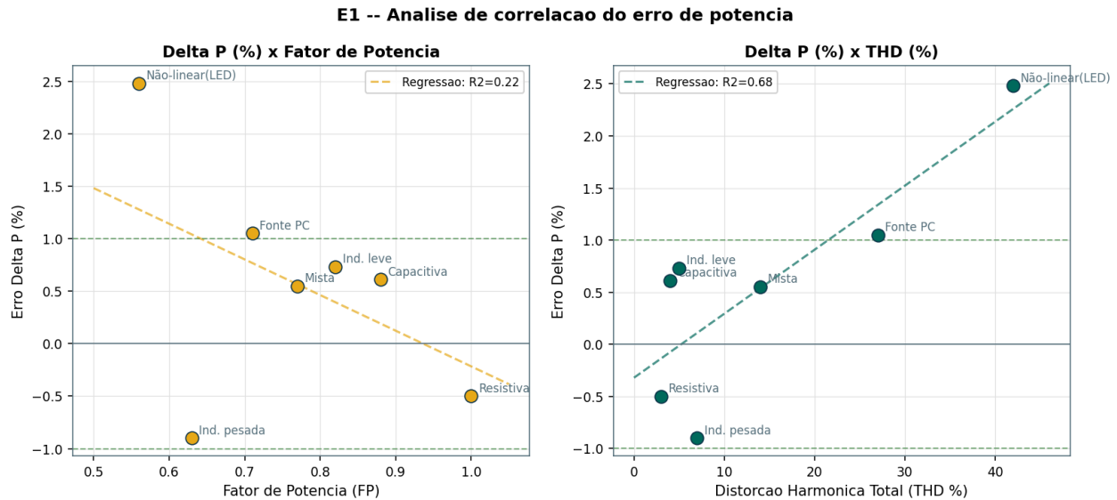
Figura 3 – Diagramas de dispersão: \Delta P(\%) \times FP (esquerda) e \Delta P(\%) \times THD\% (direita). Linhas tracejadas mostram regressão linear com R^2 indicado.
