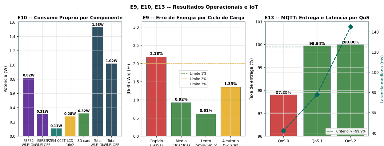
Figura 10 – Da esquerda para a direita: (1) consumo próprio por componente do sistema; (2) erro |\Delta Wh| por ciclo de carga (E9); (3) taxa de entrega e latência MQTT por nível de QoS (E13).
