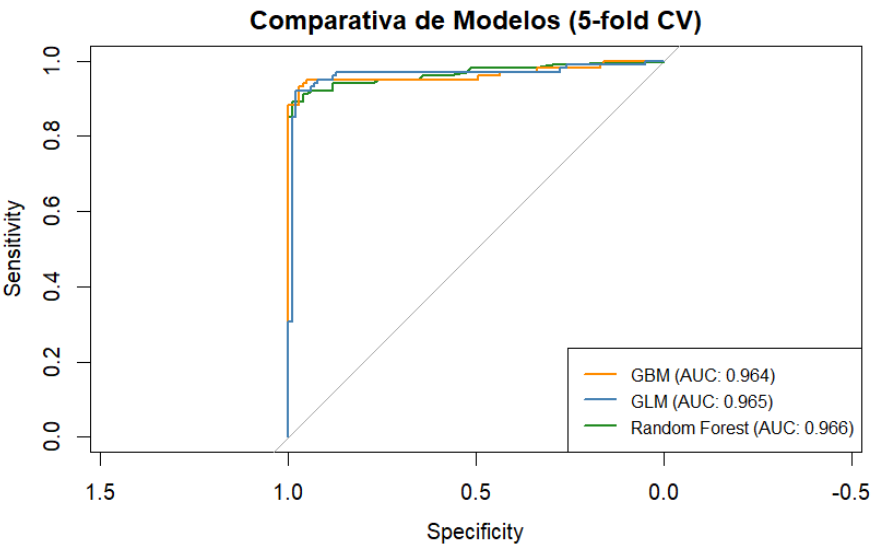
Figura 4.1: Curvas ROC conjuntas ( pooled ) obtenidas tras la validación cruzada. Se observa un empate técnico absoluto entre las tres aproximaciones matemáticas al evaluar el conjunto global de predicciones.
