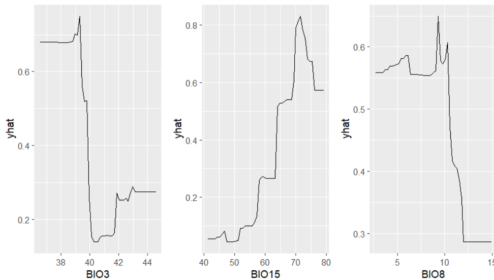
Figura 4.6: Curvas de Dependencia Parcial (PDP) del algoritmo Random Forest . Se observan transiciones abruptas en forma de escalón, típicas de arquitecturas basadas en árboles profundos.
