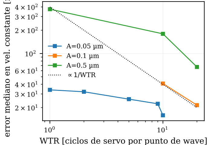
(b) WTR: el único knob de velocidad v = \Delta x / (WTR \times 40 \mu\text{s})
