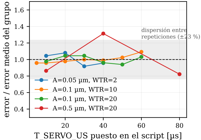
(a) T_SERVO_US: variable nula (no se le manda al controlador)
