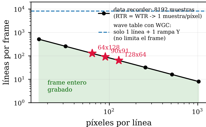
(a) los dos presupuestos son distintos
