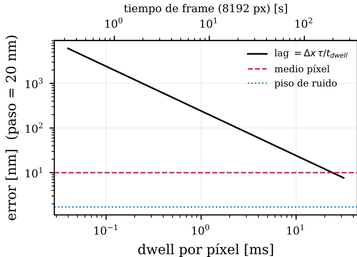
(b) por qué hay que CORREGIR el lag, no esperarlo
