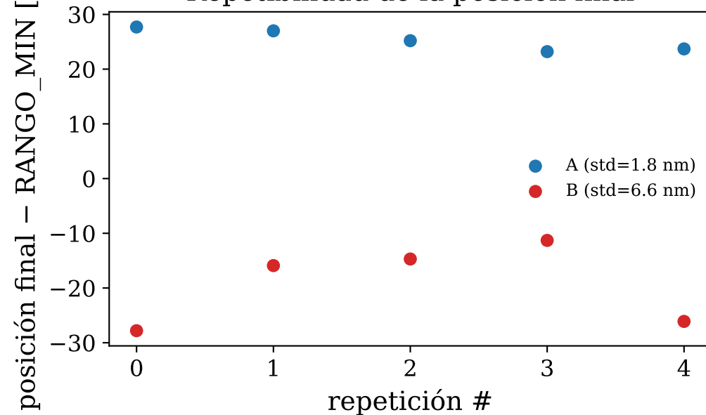
Repetibilidad de la posición final
