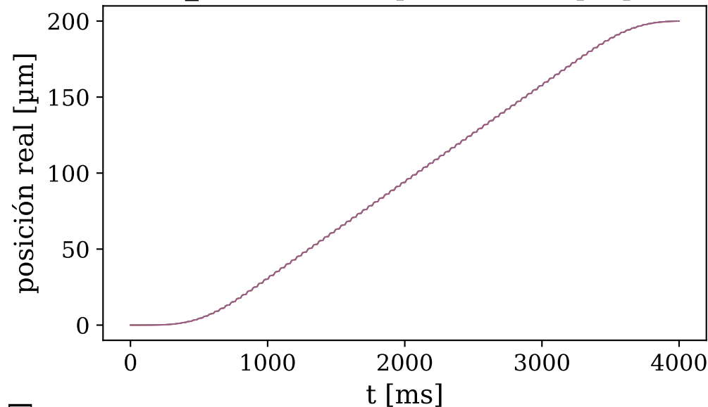
B) WAV_LIN (ida) — repeticiones superpuestas
