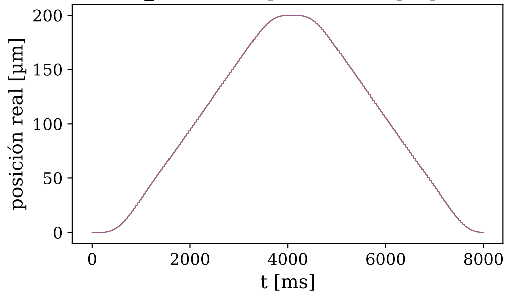
A) WAV_RAMP — repeticiones superpuestas
