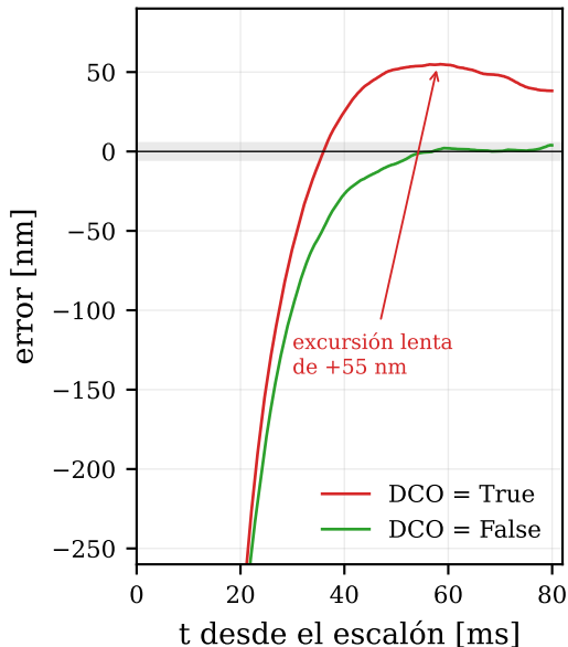
(a) par controlado 02/09 escalón 2 \mu\text{m} , misma ventana
