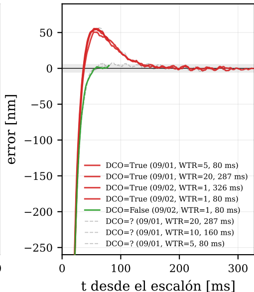
(b) todas las corridas de 2000 nm (los dos días, todos los WTR)
