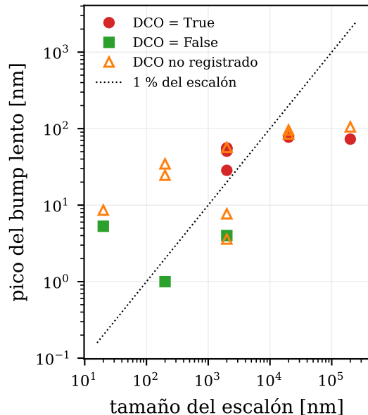
(c) el bump es ~50-100 nm ABSOLUTOS, casi independiente del escalón
