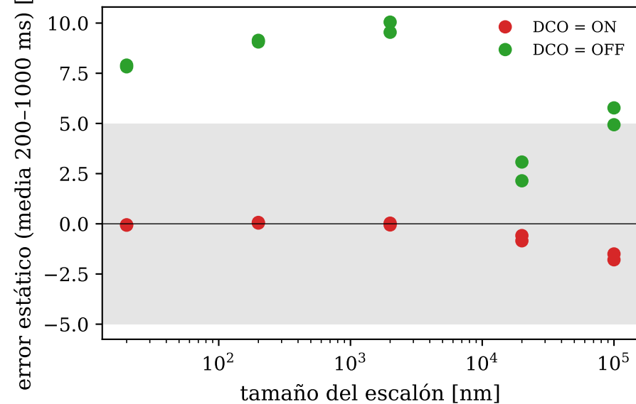
(c) POR QUÉ con DCO apagado no asienta a \pm 5 nm: queda un offset estático que DCO anula
