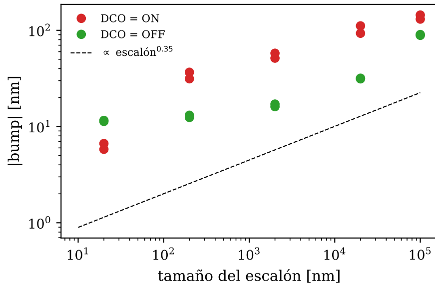
(b) el bump SÍ crece con el escalón (sublineal)
