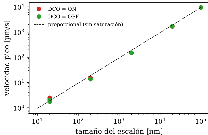
(d) sin límite de slew hasta 100 \mu\text{m}
