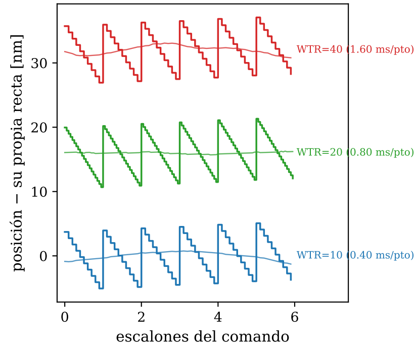
(a) seis escalones: el comando es un diente de sierra de \pm dx/2 (escalonado) y la medida sale plana (línea fina)
