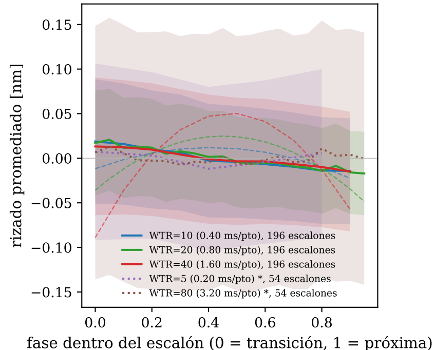
(b) escalón promedio: medido (llena) vs simulado con \tau (rayada)
