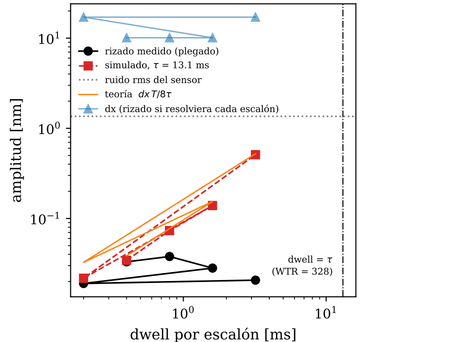
(c) el rizado nunca se acerca a dx : la platina no ve los escalones
