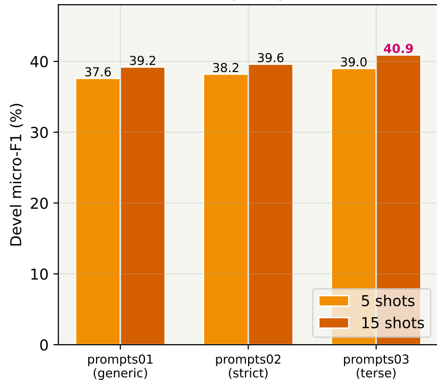
Micro-F1 — prompt × shots
