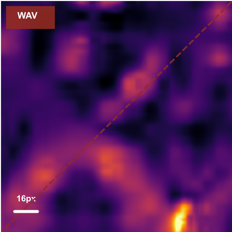
Wavelet · db4
