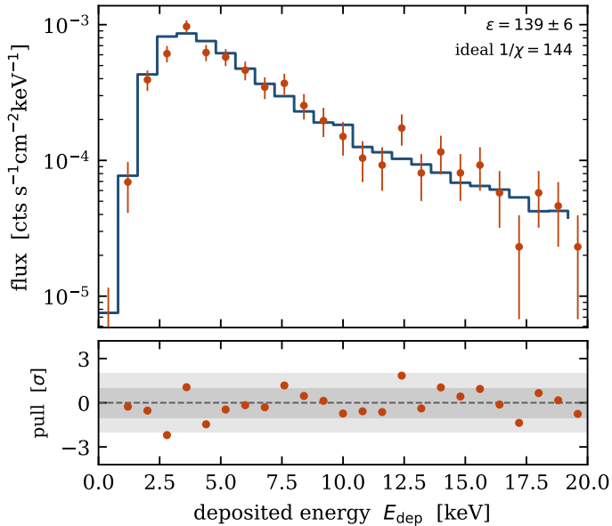
(b) SRON XFDM – Detector 1, TES array
