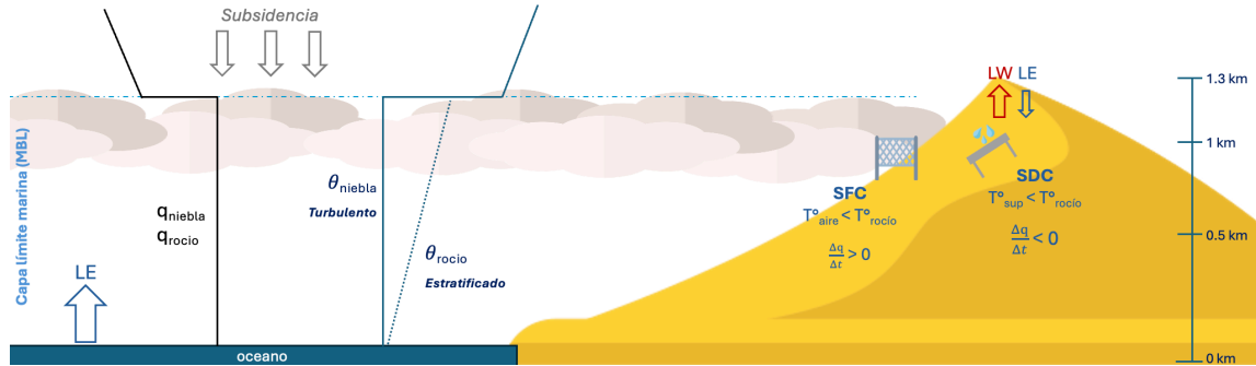
Figura 1: Esquema conceptual de la termodinámica de la niebla y el rocío en el desierto costero de Atacama. La niebla se asocia a la advección de un estratocúmulo marino (Sc) sobre una capa límite marina (MBL) comparativamente bien mezclada, coronada por una inversión térmica reforzada por la subsidencia, y se colecta con un colector estándar de niebla (SFC) donde la nube intersecta la ladera ( T_{\text{aire}} \leq T_{\text{rocío}} ; \Delta q / \Delta t \geq 0 ). El rocío se forma por enfriamiento radiativo nocturno de la superficie ( T_{\text{sup}} \leq T_{\text{rocío}} ), con emisión de onda larga (LW) y un flujo de calor latente (LE) dirigido hacia la superficie, y se colecta con un colector estándar de rocío (SDC) en la cima ( \Delta q / \Delta t < 0 ). Las temperaturas potenciales ilustran el contraste de estabilidad, una capa más mezclada (turbulenta) y más estratificada, mientras que la humedad específica ( q ) permanece comparable entre ambos regímenes. Figura de elaboración propia, adaptada de la Figura 1 de Lobos-Roco et al. (2024).
