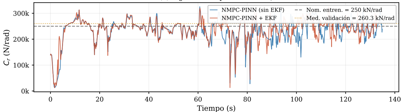
(b) Rigidez de esquina trasera C_r
