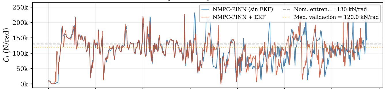
(b) Rigidez de esquina trasera C_r
