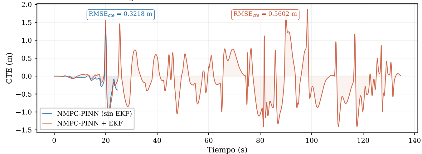
Error de seguimiento lateral: NMPC-PINN sin EKF vs NMPC-PINN + EKF
