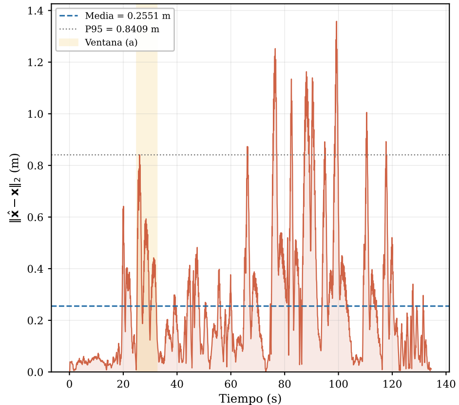
(b) Error de estimación de posición EKF
