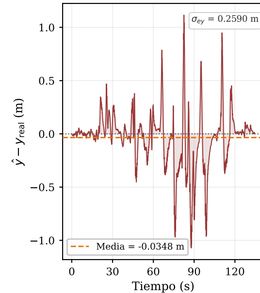
(e) Error de estimación y
