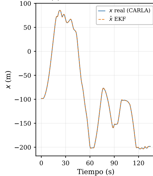
(b) Posición x: real vs. EKF
