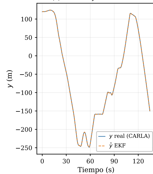
(c) Posición y: real vs. EKF
