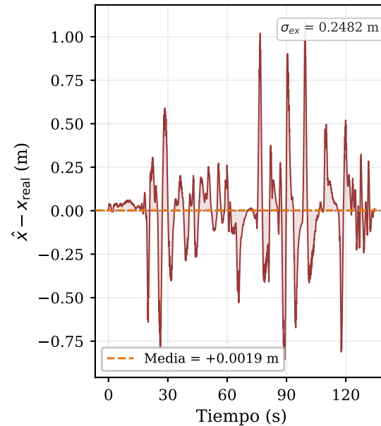
(d) Error de estimación x
