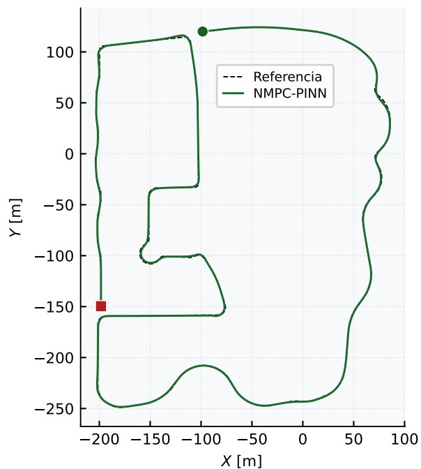
(d) NMPC-PINN (RMSE = 0.4486 m)
