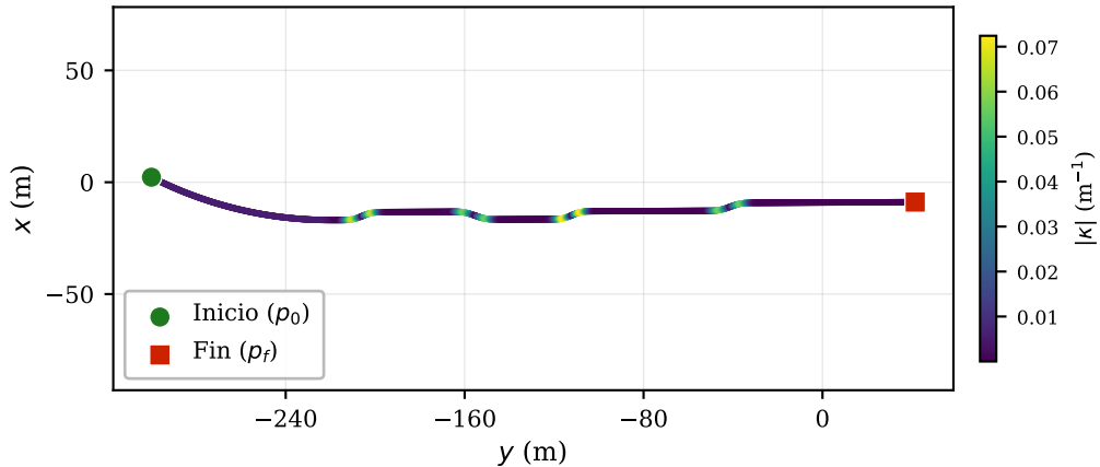
Escenario 2: maniobra de cambios de carril a alta velocidad
