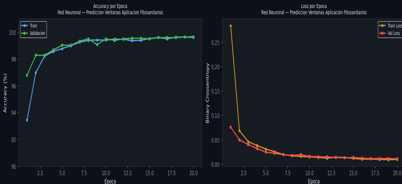
Fig. 5 — Curvas de entrenamiento de la red neuronal para prediccion de ventanas de aplicacion de fitosanitarios: accuracy (izq.) y loss (der.) por epoca. Convergencia estable. Accuracy final en validacion: 99.65%.
