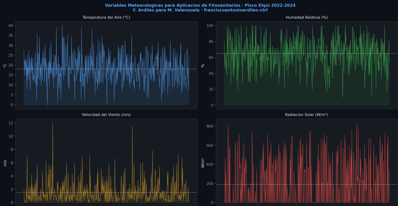
Fig. 1 — Serie temporal de variables meteorologicas en Pisco Elqui (muestra 500 registros). La velocidad del viento (naranja) es el factor critico para decidir si aplicar fitosanitarios.
