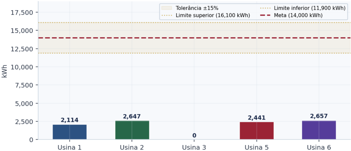
Geração Mensal por Usina — Abril/2026
