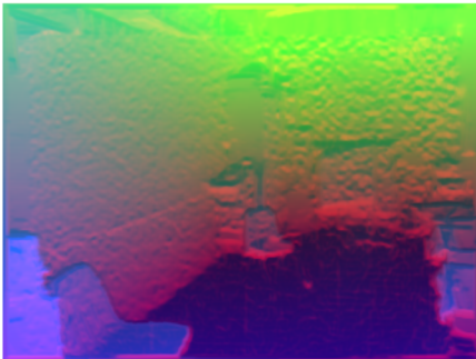
CMAAttention
