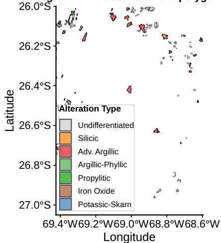
b) Region III — Atlas Metalífero polygons
