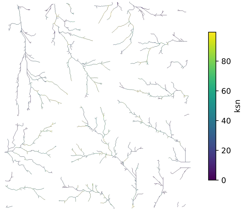
ksn map (Wobus 2006)
