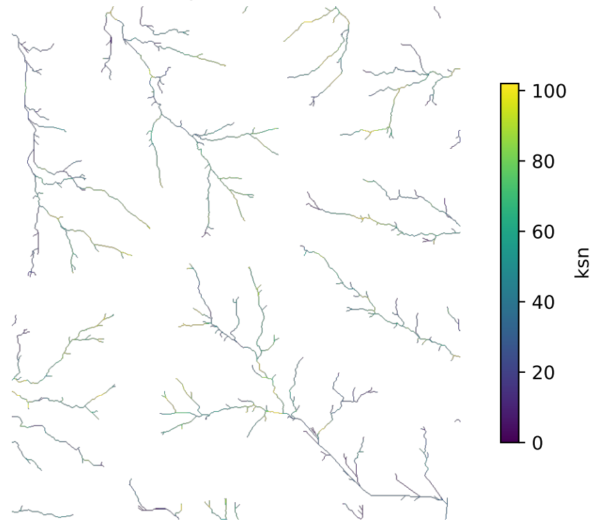
ksn map (Wobus 2006)
