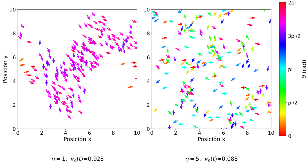
Figura 1: Configuraciones del modelo de Vicsek para \rho = 2 y t = 2000 . Panel izquierdo: \eta = 1 . Panel derecho: \eta = 5 . El color codifica la orientación de la velocidad.
