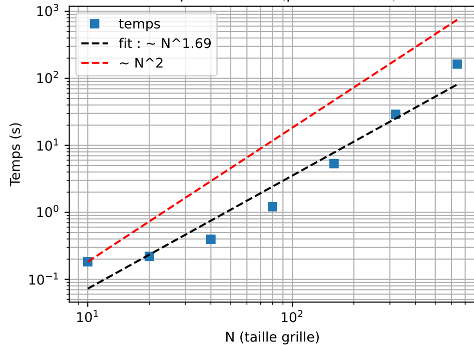
Temps de calcul (pente \approx 1.69 )
