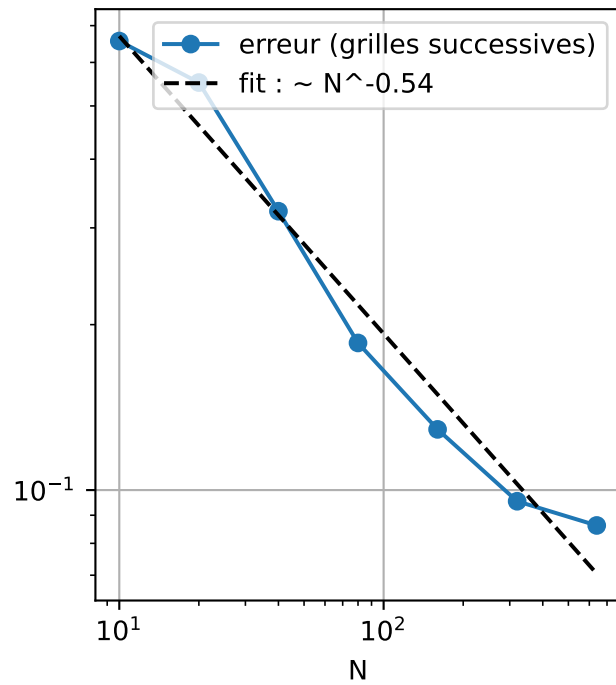
Convergence en N/benchmark, évalué par analytique
