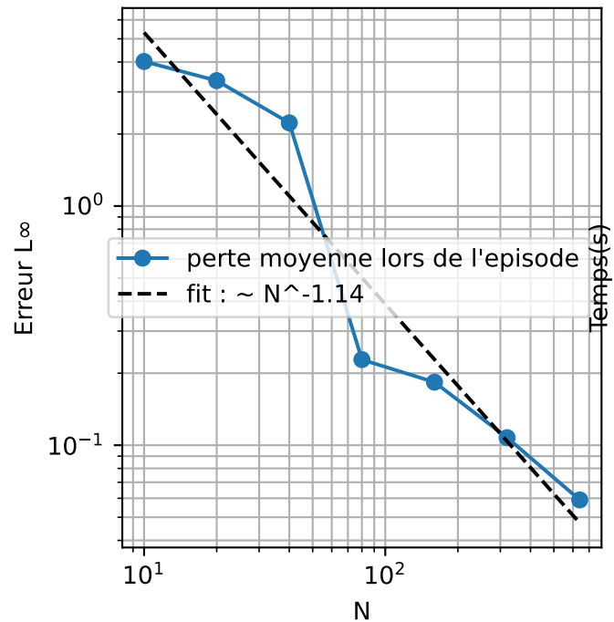
Convergence de la perte face au nombre d'épisodes
