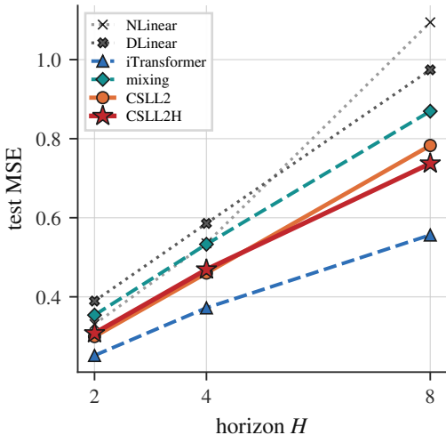
US-state influenza
