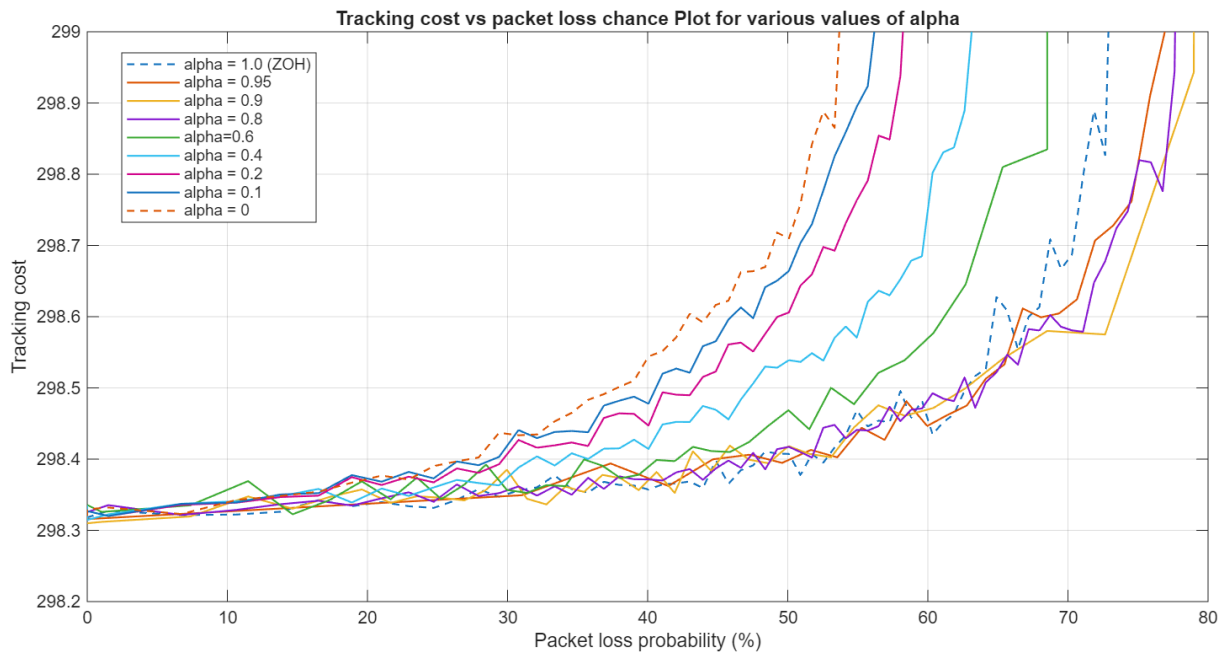
Fig. 19 – Andamento mediano del costo di tracking al variare della probabilità di perdita, valutato per vari livelli di \alpha . Risultato basato sullo svolgimento di 30 simulazioni per ogni valore di p_{loss} , della durata di 25s ciascuna.
