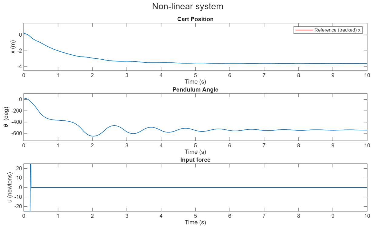
Fig. 10 - Simulazione dei sistemi - lineare e reale - a ciclo chiuso in risposta a condizioni iniziali estreme, non stabilizzabili. Specifiche simulazione: y_0 = [0.2, -0.2, 0.4, 0.8] , Guadagno K come in Fig. 8. Il controllore viene disabilitato se |\theta| > 0.8 (rad) .
