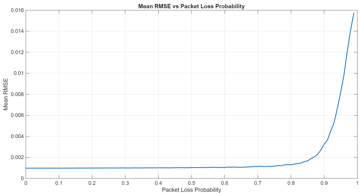
Fig. 8 – Andamento dell'RMSE medio all'aumentare della probabilità di perdita. il valore di RMSE viene calcolato mediando su un 100 episodi aleatori, per ogni valore della probabilità di perdita di pacchetti.
