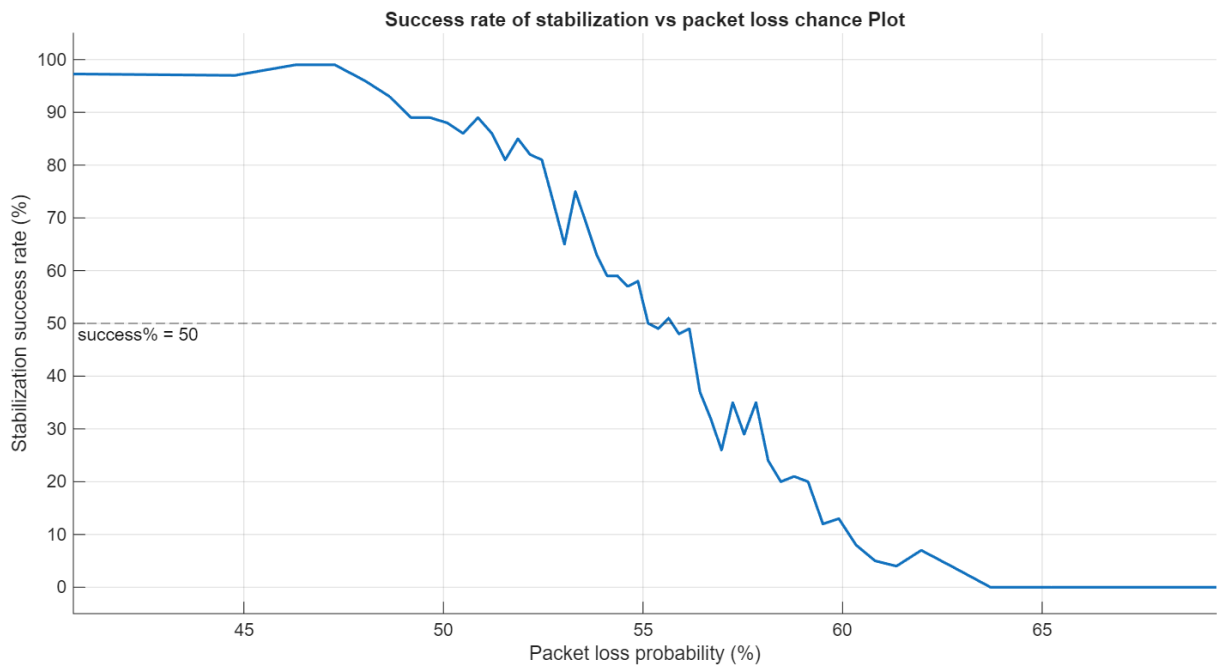
Fig. 14 - Percentuale di successo nella stabilizzazione al variare della probabilità di perdita. Ogni punto è misurato mediando il successo su un pool di 100 simulazioni, dalla durata di 25 s ciascuna. Nessuna policy di compensazione attiva.
