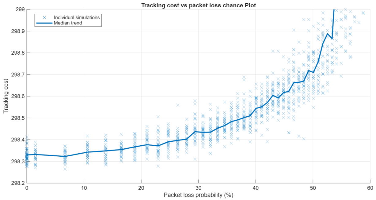
Fig. 13 - Andamento mediano e individuale (per simulazione) del costo di tracking al variare della probabilità di perdita. Risultato basato sullo svolgimento di 100 simulazioni per ogni valore di p_{loss} , della durata di 25s ciascuna. Nessuna policy di compensazione attiva.
