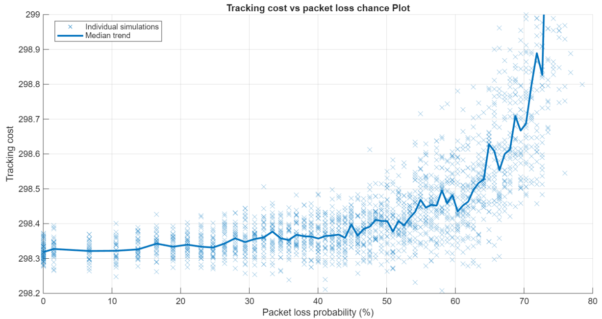
Fig. 15 - Andamento mediano e individuale (per simulazione) del costo di tracking al variare della probabilità di perdita, con policy di ZOH ( \alpha = 1 ). Risultato basato sullo svolgimento di 100 simulazioni per ogni valore di p_{loss} , della durata di 25s ciascuna.
