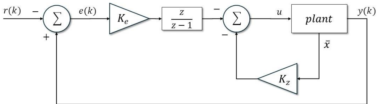
Fig. 11 - Diagramma a blocchi del controllore tempo-discreto, costruito con IMD.
