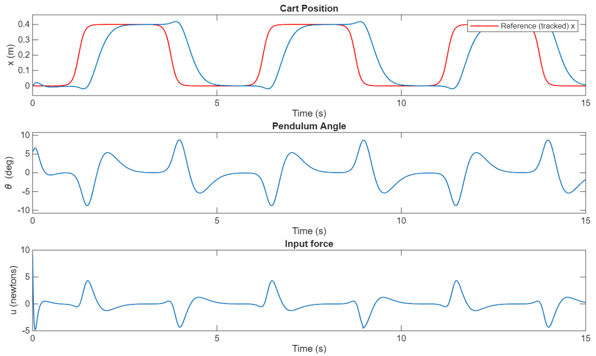
Fig. 12 – Sistema a ciclo chiuso con integratore per tracciamento del gradino. Specifiche di simulazione: y_0 = [0; 0.2; 0.1; -0.1] ; Parametri del riferimento x_{ref} : T = 5 , k = 5 , A = 0.2 . Gain del controllore: K_z = [-1092.95, -315.95, 638.34, 98.460] , K_e = -8.83 .
