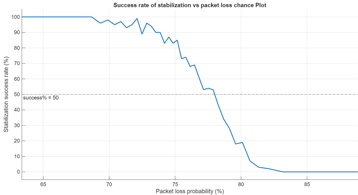
Fig. 16 - Percentuale di successo nella stabilizzazione al variare della probabilità di perdita, con policy di ZOH ( \alpha = 1 ). Ogni punto è misurato mediando il successo su un pool di 100 simulazioni, dalla durata di 25 s ciascuna.
