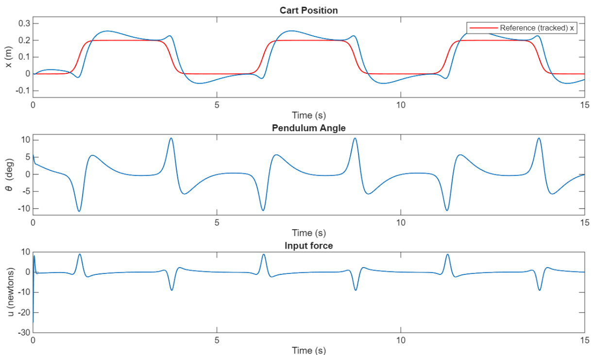
Fig. 2 - Stabilizzazione con controllore PID
