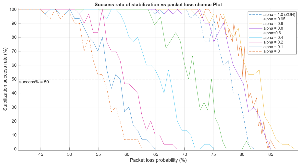
Fig. 17 - Percentuale di successo nella stabilizzazione al variare della probabilità di perdita, per vari livelli di \alpha . Ogni punto è misurato mediando il successo su un pool di 30 simulazioni, dalla durata di 25 s ciascuna. Ogni curva è composta da 100 campioni, distribuiti in maniera adattiva attorno al valore di p_{loss} di interesse (in cui si concentra la maggiore variazione).
