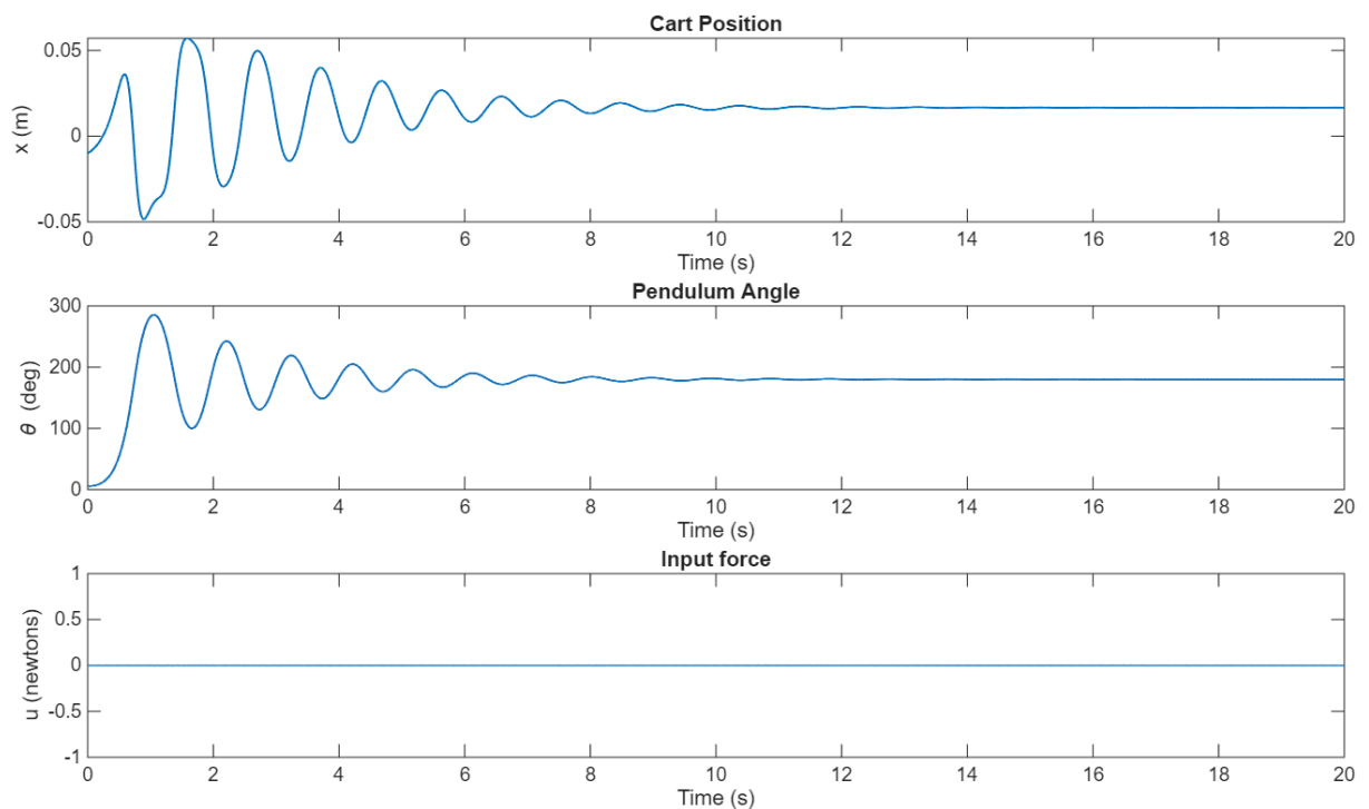
Fig. 1 - Simulazione preliminare senza controllo Specifiche simulazione: y_0 = [-0.01; 0.02; 0.1; -0.1] .
