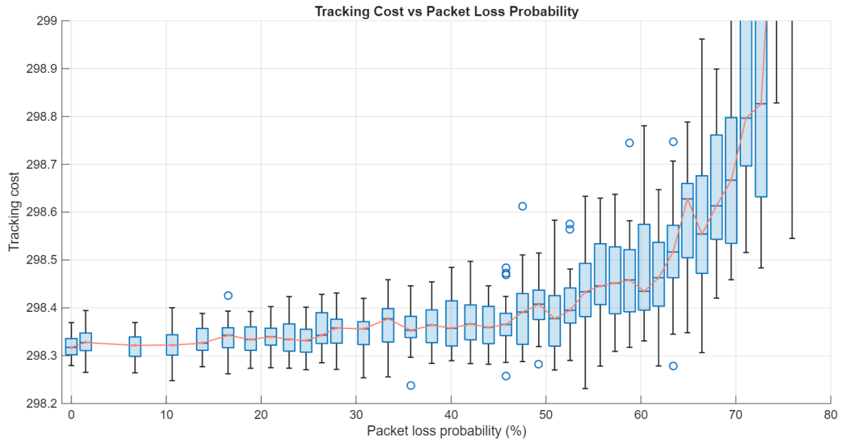
Fig. 17 – Boxchart del costo di tracking al variare della probabilità di perdita, con policy di ZOH ( \alpha = 1 ). Risultato basato sullo svolgimento di 100 simulazioni per ogni valore di p_{loss} , della durata di 25s ciascuna.
