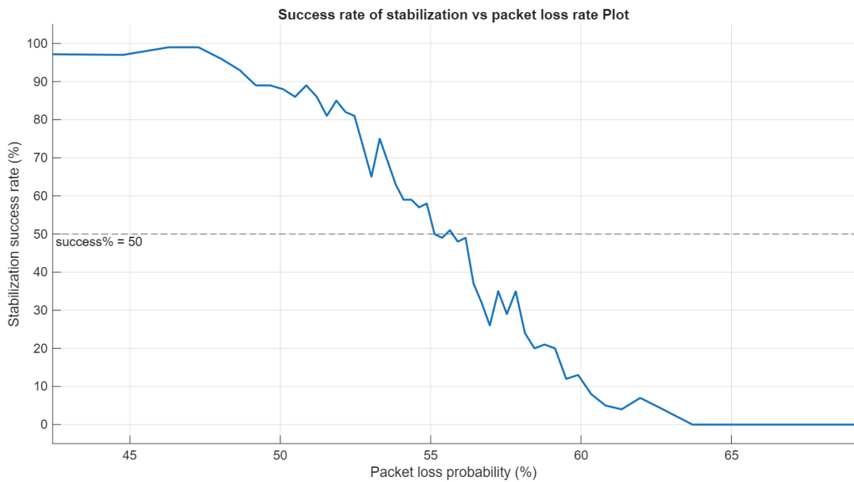
Fig. 16 – Percentuale di successo nella stabilizzazione al variare della probabilità di perdita. Ogni punto è misurato mediando il successo su un pool di 100 simulazioni, dalla durata di 25 s ciascuna. Nessuna policy di compensazione attiva.
