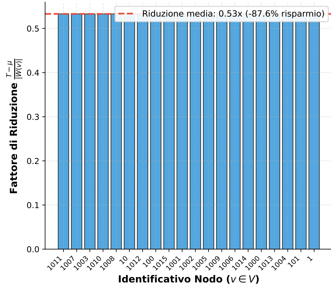
Efficacia del Pruning Temporale per Nodo
