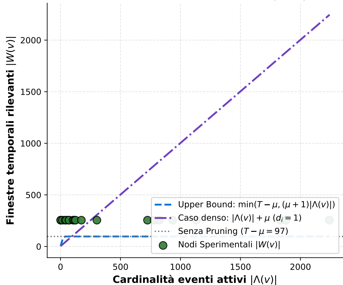
Conformità ai Bound Teorici di |W(v)|
