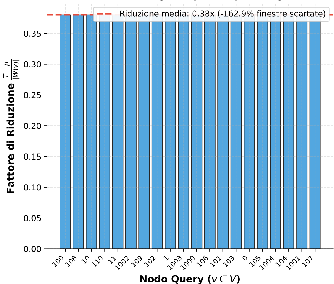
Efficacia del Pruning Temporale per Singolo Nodo
