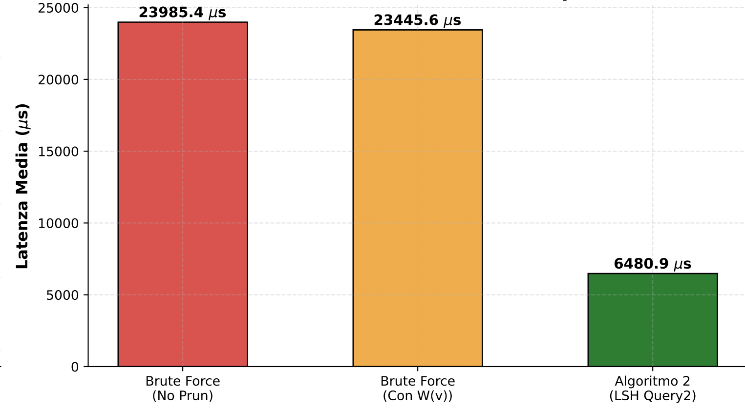
(B) Benchmark Latenza di Query
