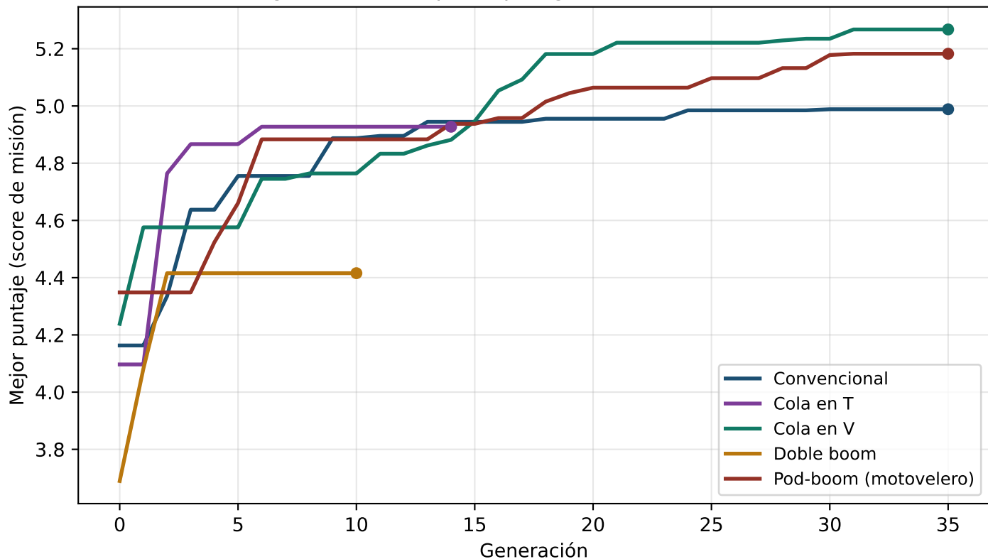
Convergencia del GA por topología -- corrida del 2026-09-18
