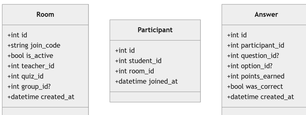
Figura 6.8: Entidades y atributos del módulo de sesiones.
