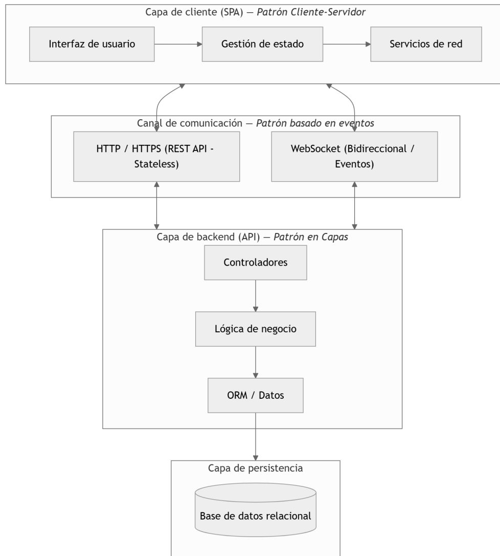
Figura 6.3: Esquema de la arquitectura global del sistema.
