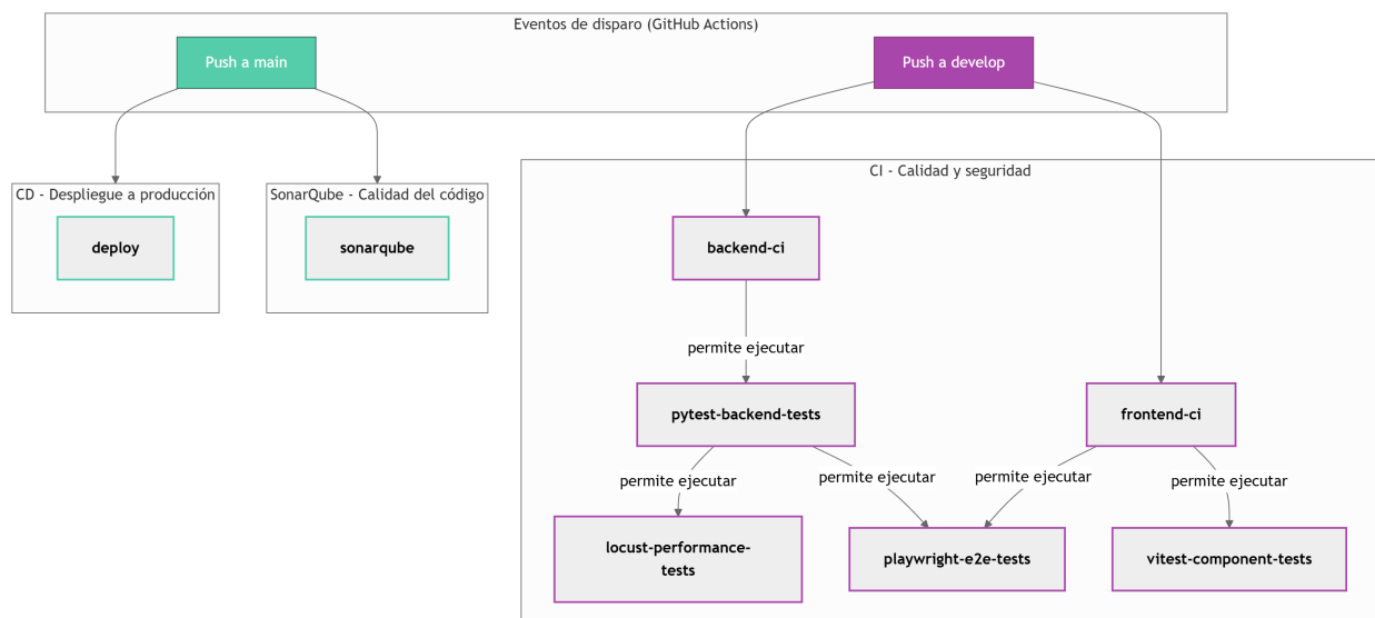
Figura 7.4: Estructura del pipeline de CI/CD
