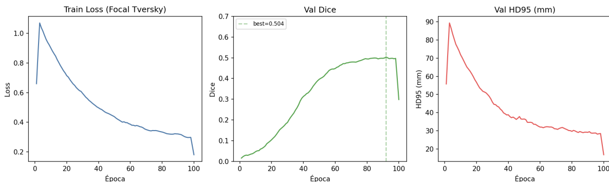
Figura 2: Curvas de entrenamiento y validación: pérdida Focal Tversky, Dice y HD95.
