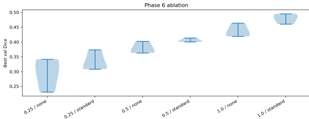
Figura 1: Distribución del Dice Score por fracción de datos y régimen de aumentación.
