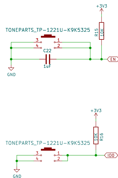
Strapping IO
