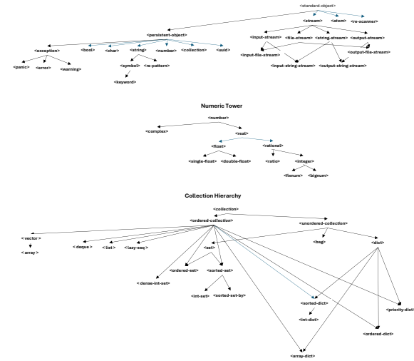
Fig. 1. FOL Type Hierarchy
