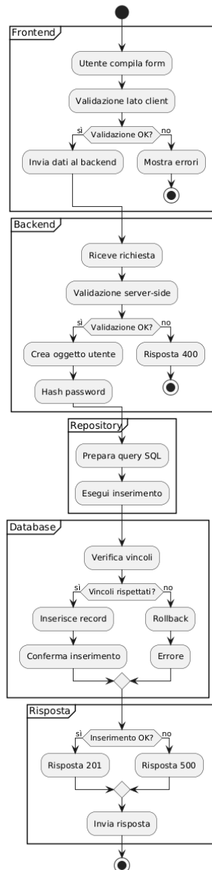
Diagramma di Attività - Inserimento Nuovo Utente
