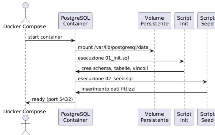
Figure 3: Diagramma di sequenza database.
