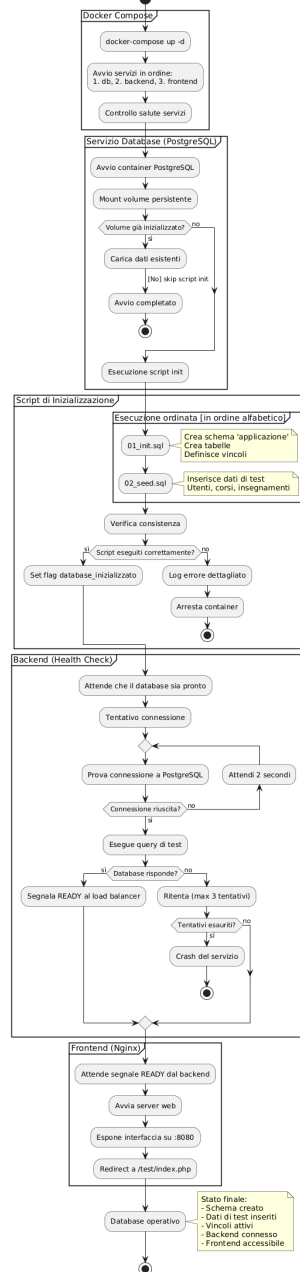
Diagramma di Attività - Inizializzazione Database con Docker
