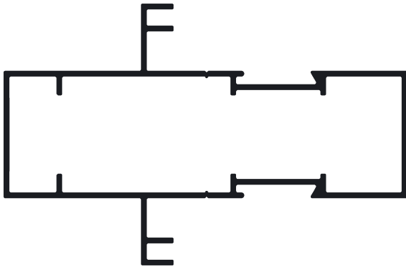
AR5-1034 Travesaño paño fijo 0,930 kg/m
