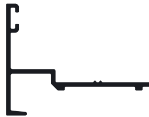
AR5-1045 Doble contacto 0,287 kg/m
