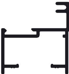
AR5-1513 Marco paño fijo chico 0,383 kg/m
