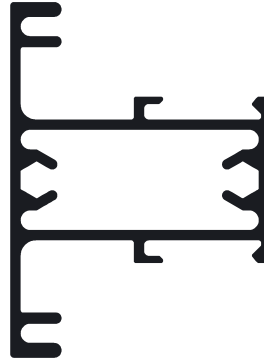
AR5-1165 Travesaño angosto paño fijo 0,747 kg/m
