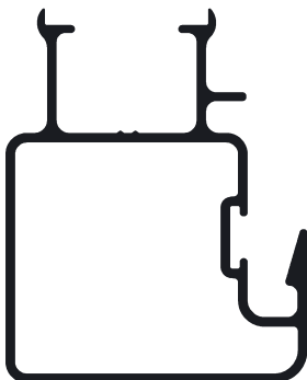
AR5-1054 Encuentro reforzado 0,600 kg/m
