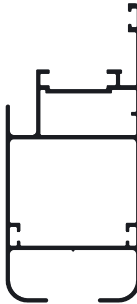
AR5-1326 Parante de puerta 0,945 kg/m
