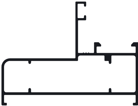
AR5-1325 Marco de puerta 0,760 kg/m
