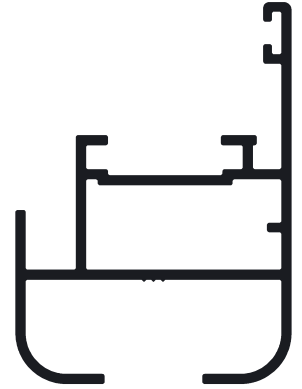
AR5-1317 Hoja batiente para vidrio simple 0,658 kg/m
