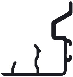
AR5-1310 Cliper (corte 90°) 0,370 kg/m
